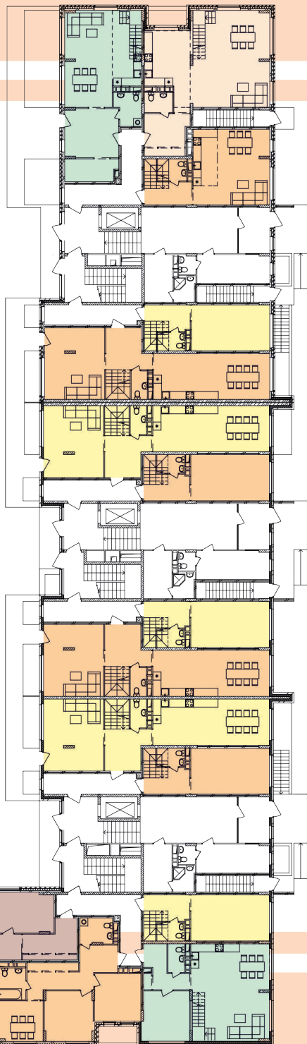
КОРПУС 2 этаж 1
