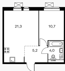
1EM4_7.2-2_S_A
